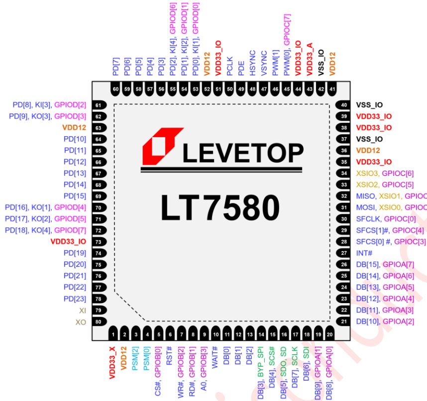
图 1-5: LT7580 引脚图 (QFN-80Pin)
