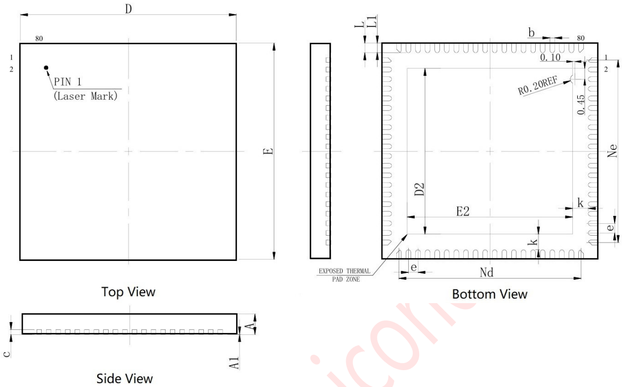
图 8-2: QFN-80Pin 外观尺寸图
