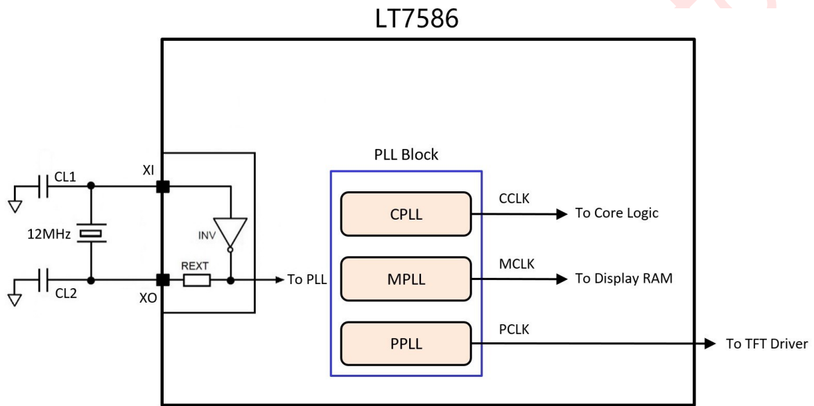
图 4-1: 3 组 PLL 电路
