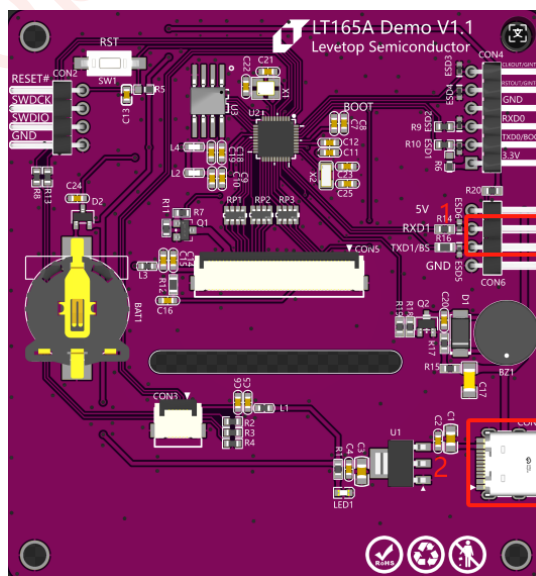
图 16-63: LT165A 开发板
