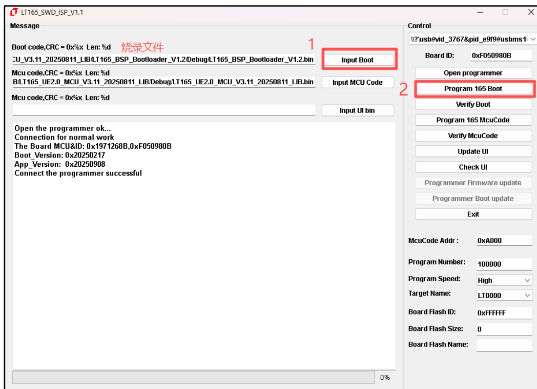
图 16-12: 导入要烧录的 Boot loader bin 文件
