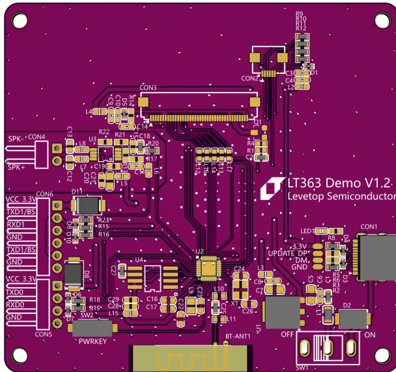
图 16-50: LT363 串口屏的开发演示板 (Demo Kit)
