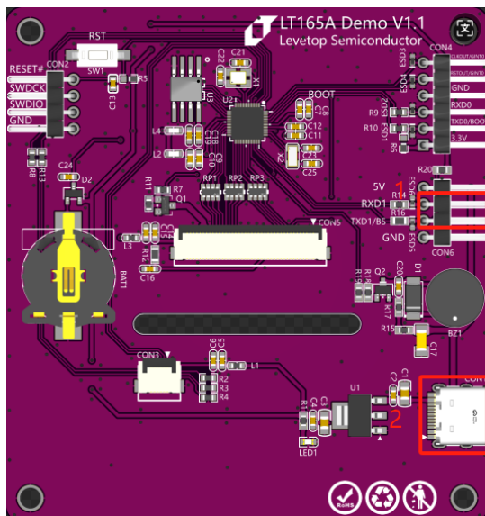
图 16-4: LT165A 开发板示意图
