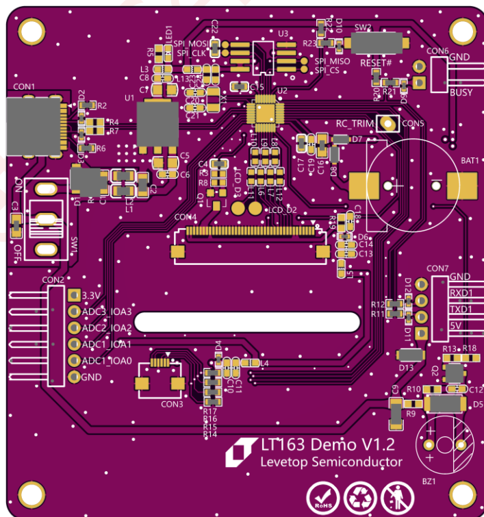
图 16-49: LT163 串口屏的开发演示板 (Demo Kit)
