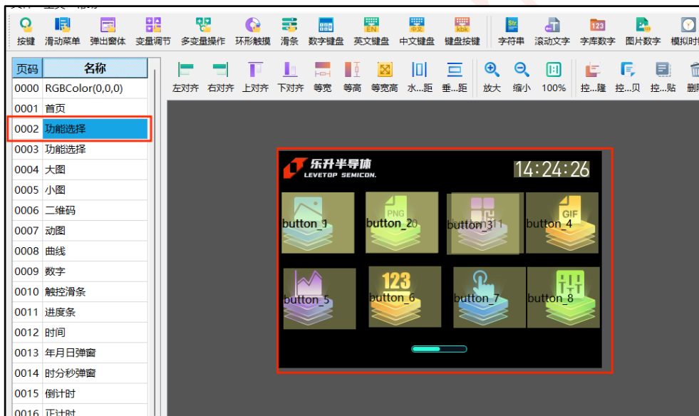
图 11-9: 示例图页面
