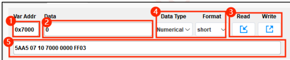
图 9-7：手动输入框
