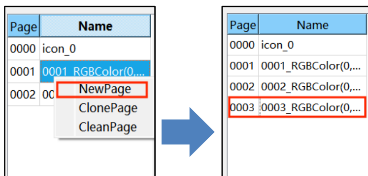
图 5-4: 添加新页
