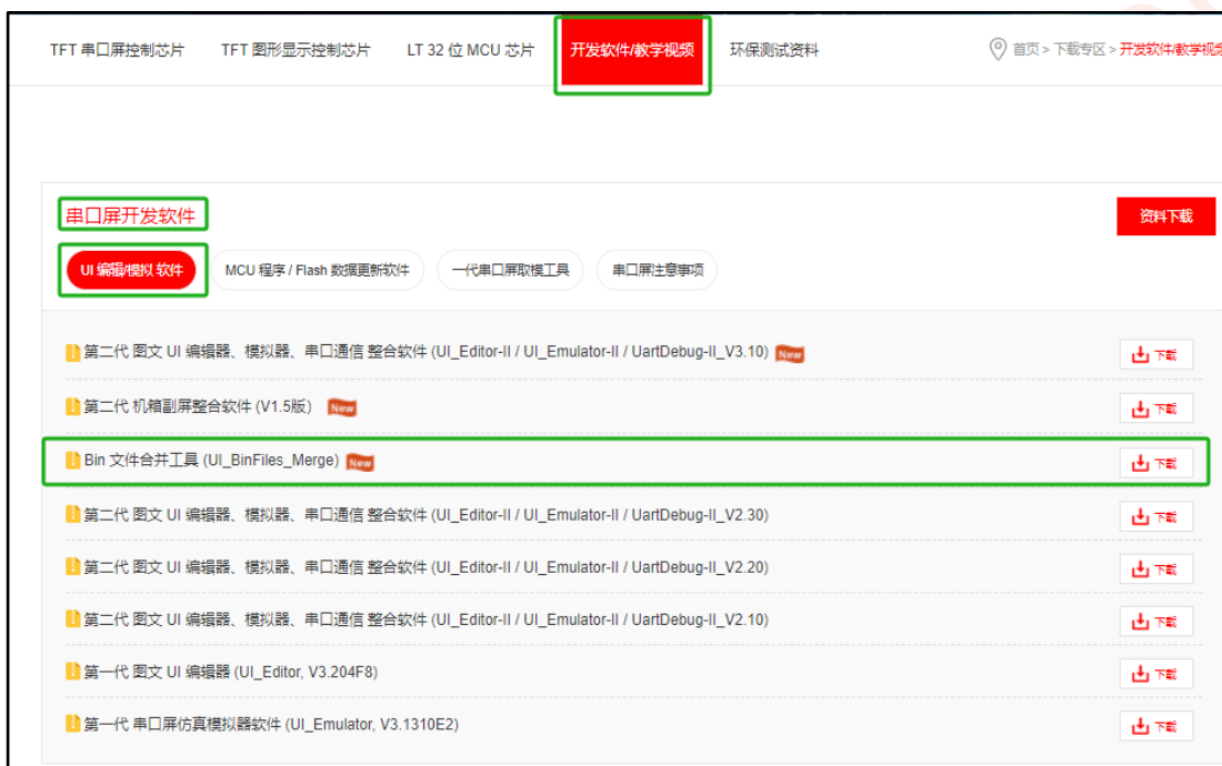
图 13-4: 下载软件包
