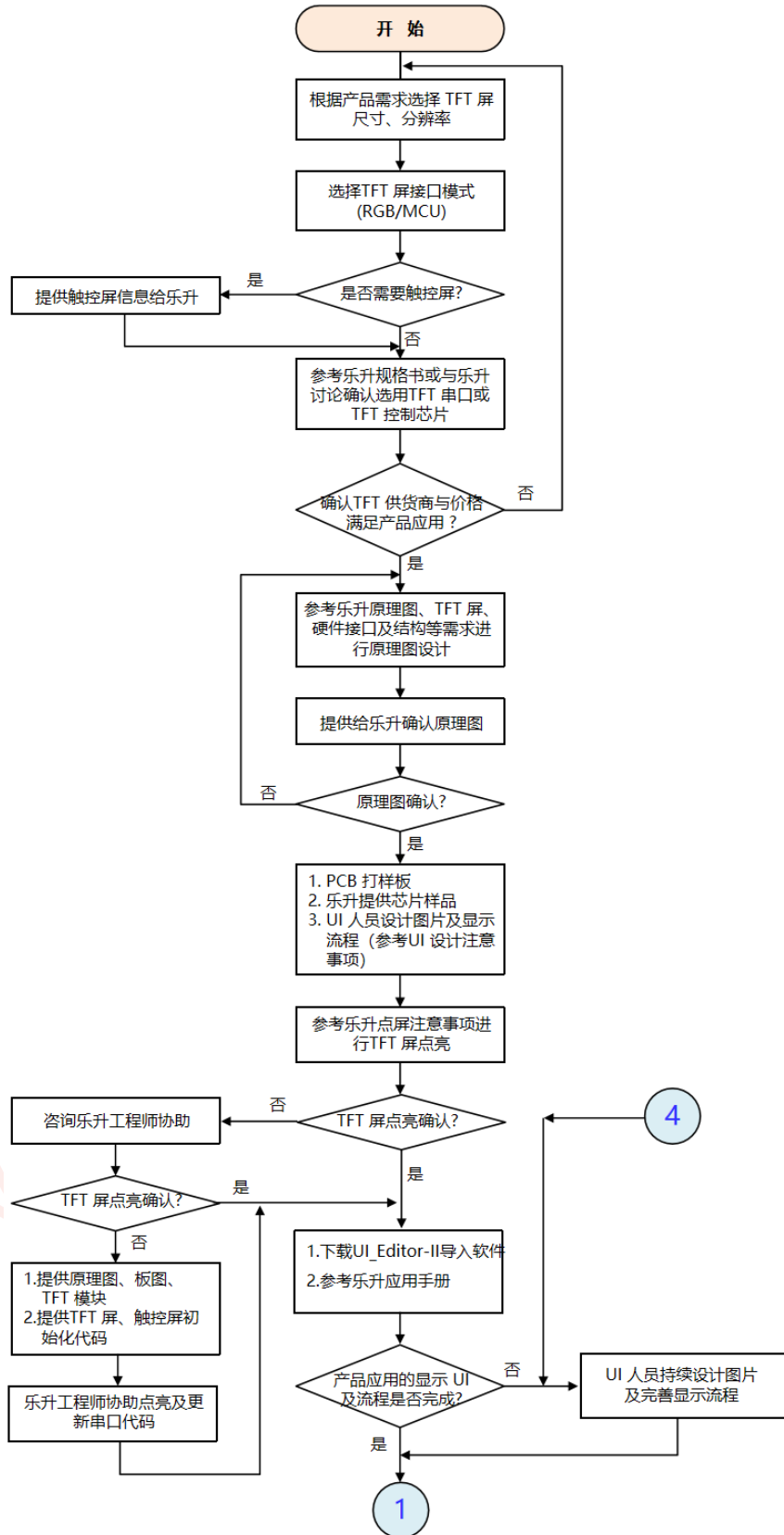
图 16-51: 开发流程 (1)
