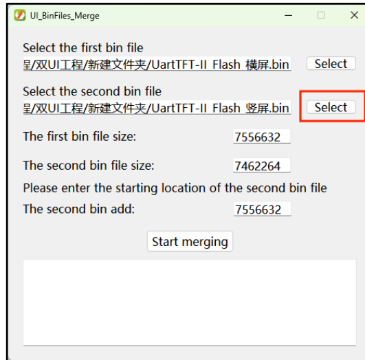
图 13-8: 添加 file2
