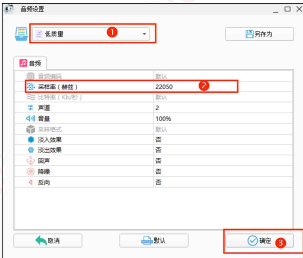
图 9-45：输出配置
