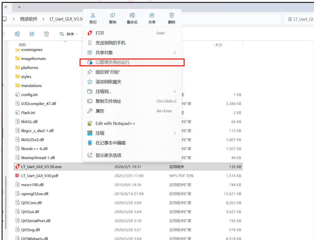
图 16-40: LT_Uart_GUI_Vx.xx.exe 软件
