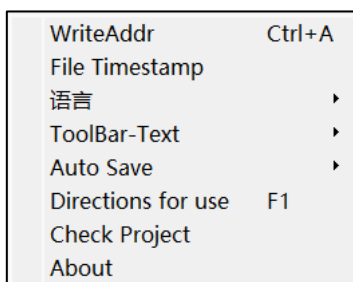
图 3-7: Help 功能
