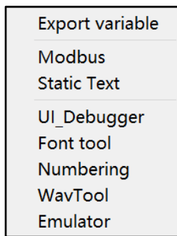
图 3-5: 工具列表
