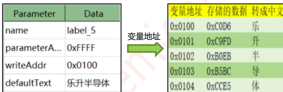
图 7-1: 变量地址内数据的储存方式
