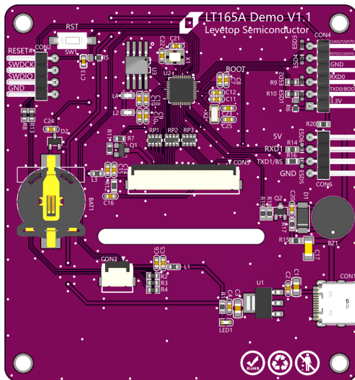
图 16-48: LT165A 串口屏的开发演示板 (Demo Kit)
