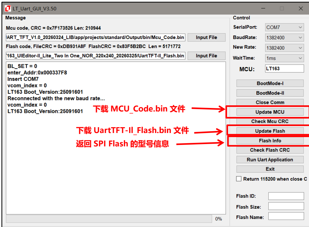
图 16-45: 烧录 UartTFT-II_Flash.bin、MCU_Code.bin 文件
