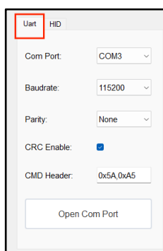
图 12-6: 选择串口
