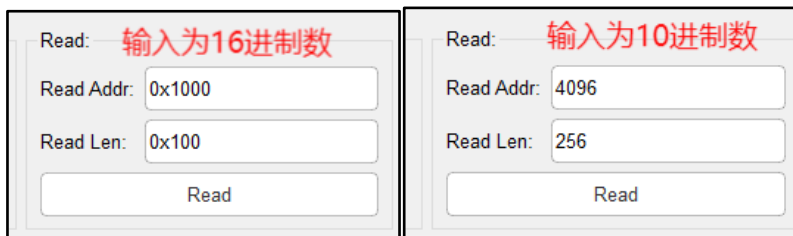
图 12-2: 地址输入框
