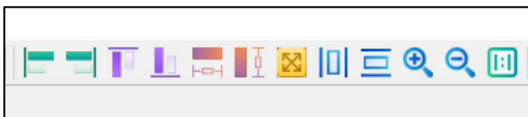
图 6-49：布局控件
