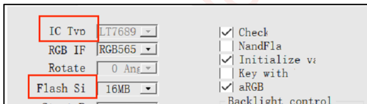
图 2-10: 错误显示
