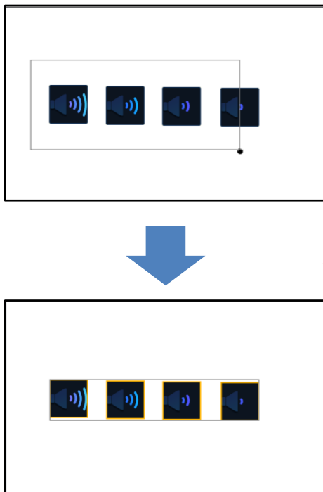
图 5-10：框选控件
