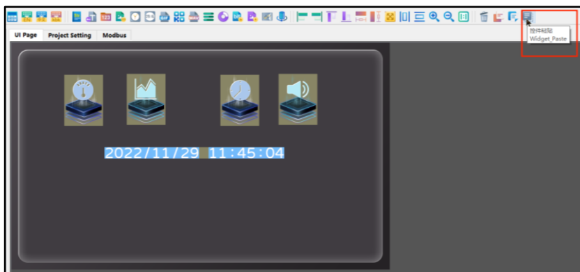
图 5-13: 粘贴控件
