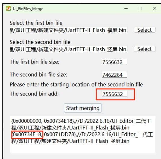
图 13-10: 合成成功
