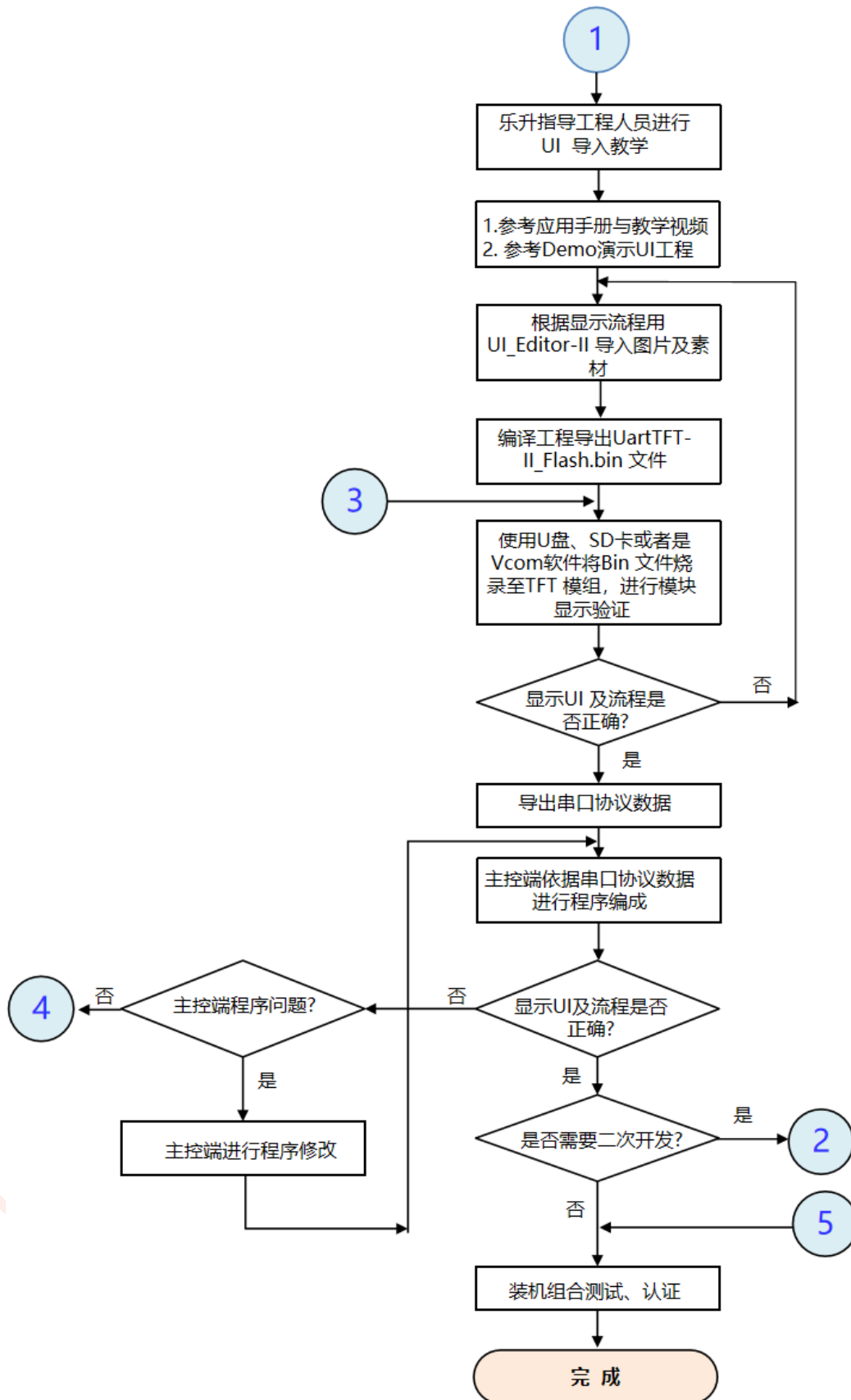
图 16-53: 开发流程 (3)
