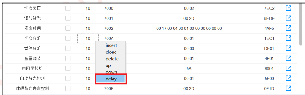
图 9-22：延时指令
