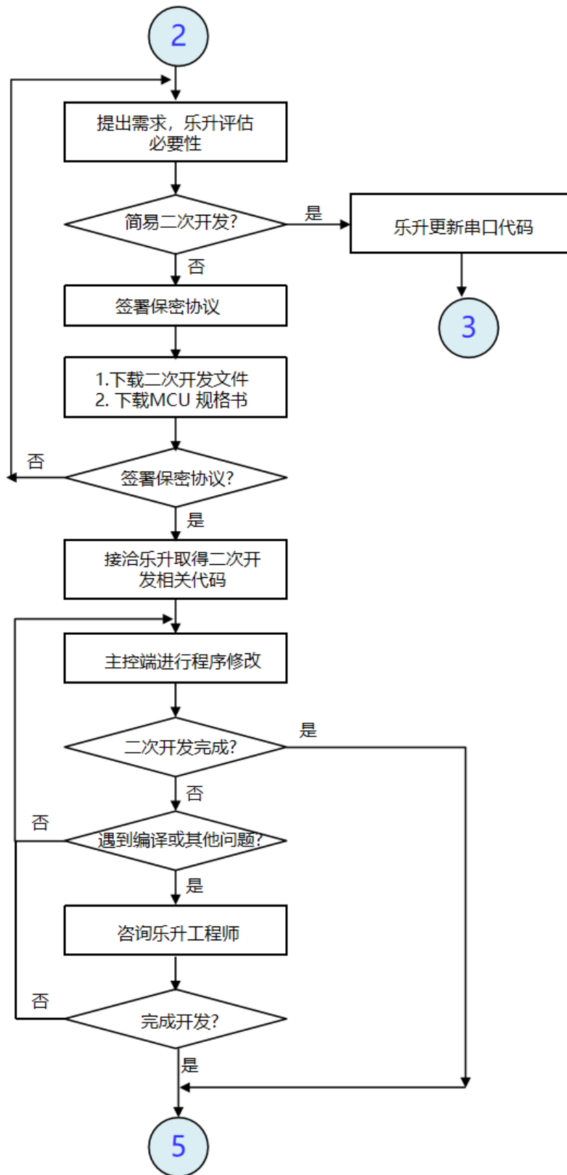
图 16-52: 开发流程 (2)
