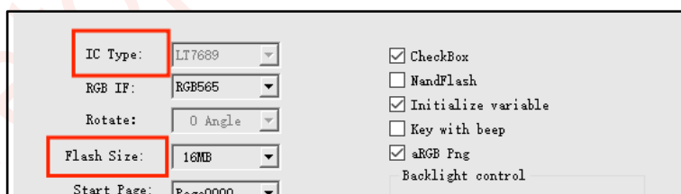
图 2-11: 正常显示
