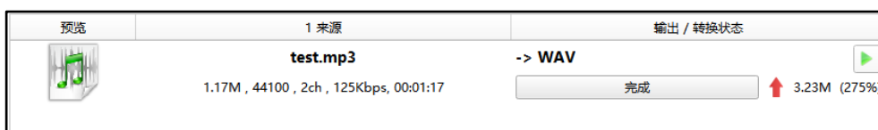
图 9-48：转换完成
