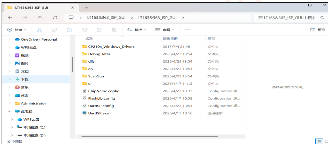
图 16-16: LT163&363_ISP_GUI 软件包
