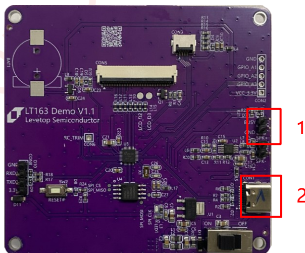
图 16-42: LT163 接线说明
