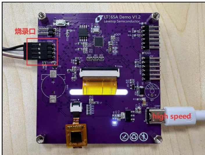
图 16-10: SWD 在线烧录接线方式
