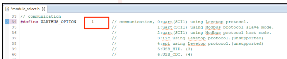
图 11-5：LT165A、LT163、LT363 选择 modbus 从机模式
