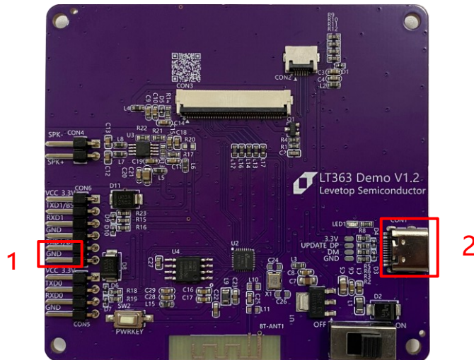
图 16-43: LT363 接线说明
