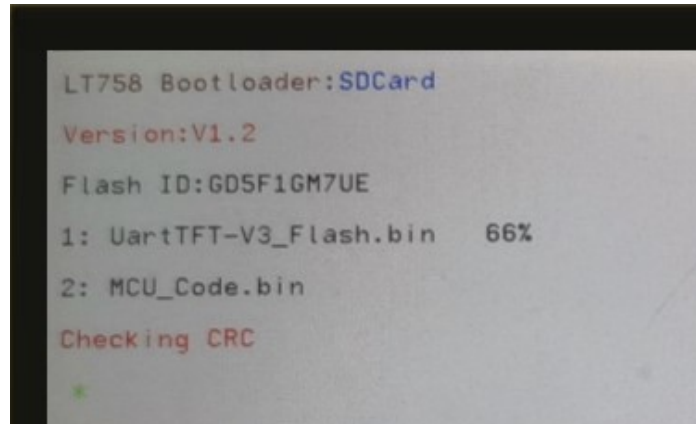
图 16-5: CRC 校验
