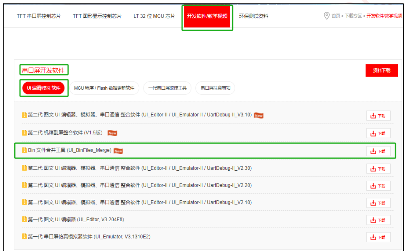
图 13-4：下载软件包
