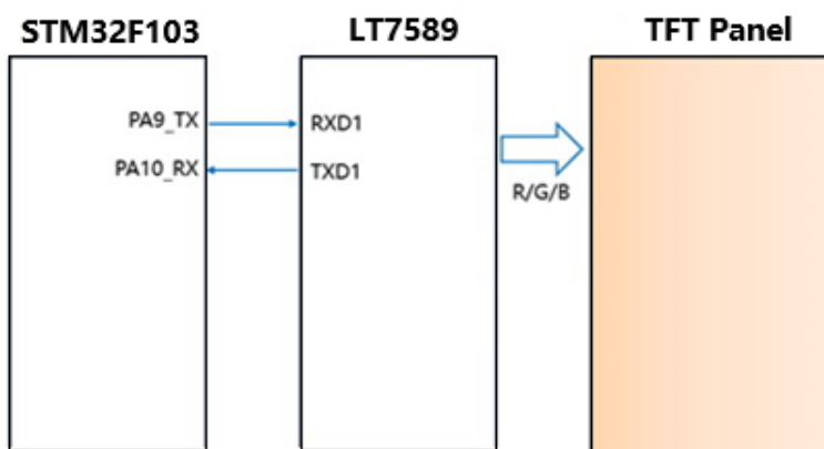
图 3-2：主控端 MCU (STM32F103RCT6)用串口与 LT7589B 串口屏芯片通讯
