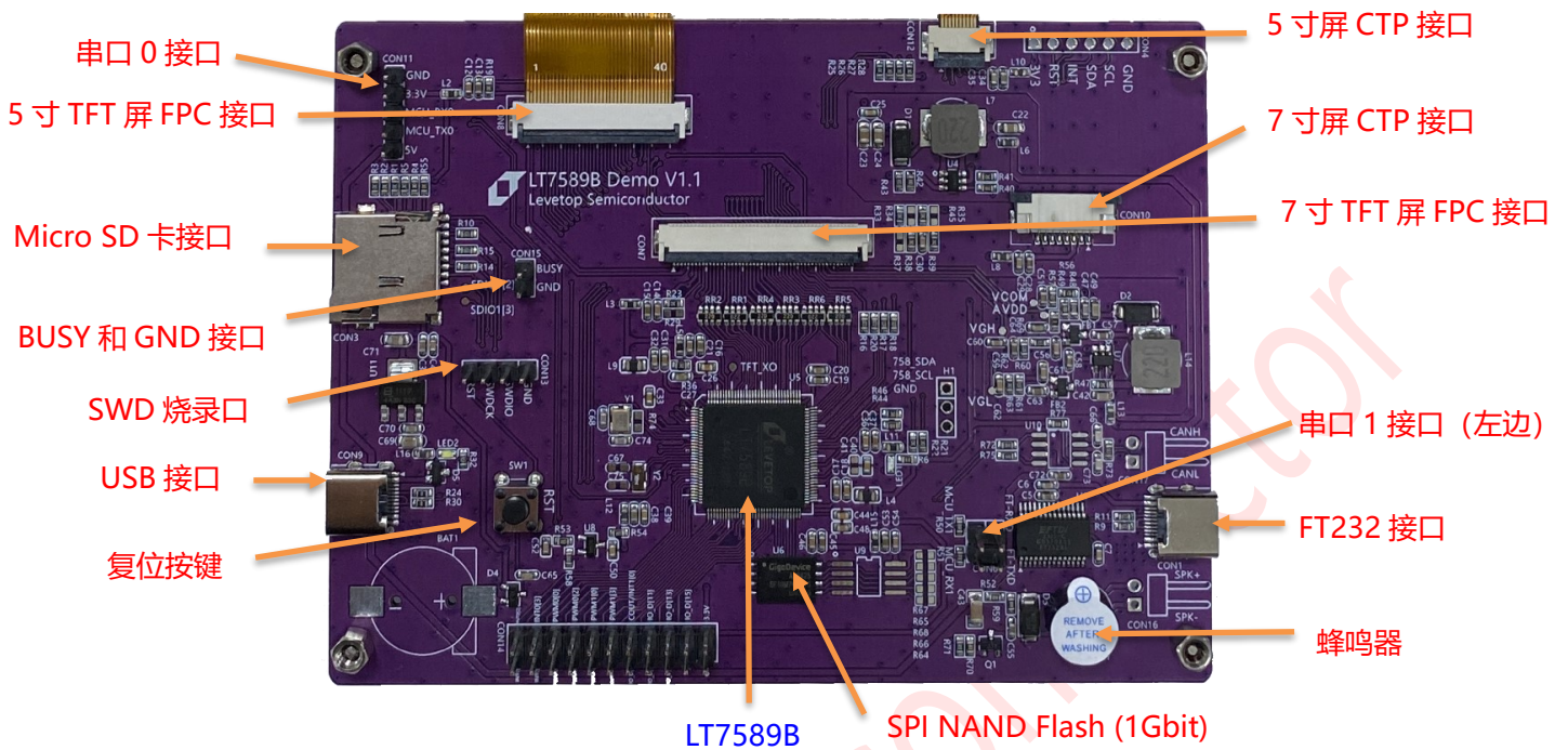
图 1-2: LT7589B 控制板主要组件与接口
