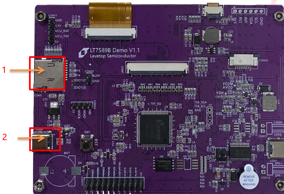
图 2-6：LT7589B 演示板示意图
