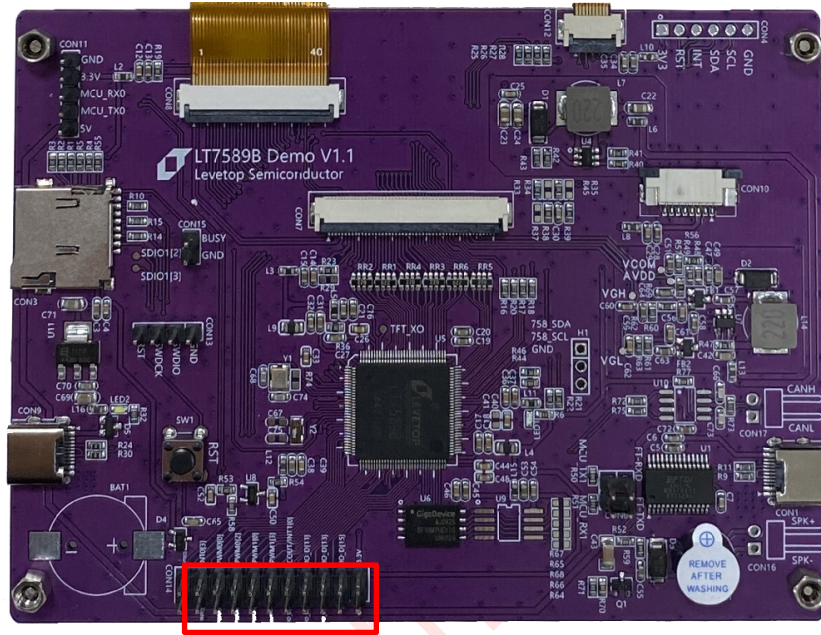
图 5-1: 模块 PCB 板上的 IO 口
