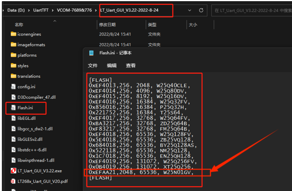
图 2-12: 添加 Flash ID
