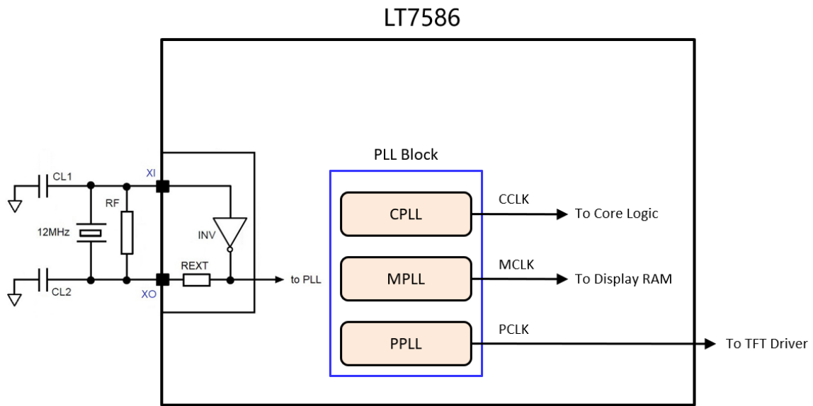
图 4-1：3 组 PLL 电路
