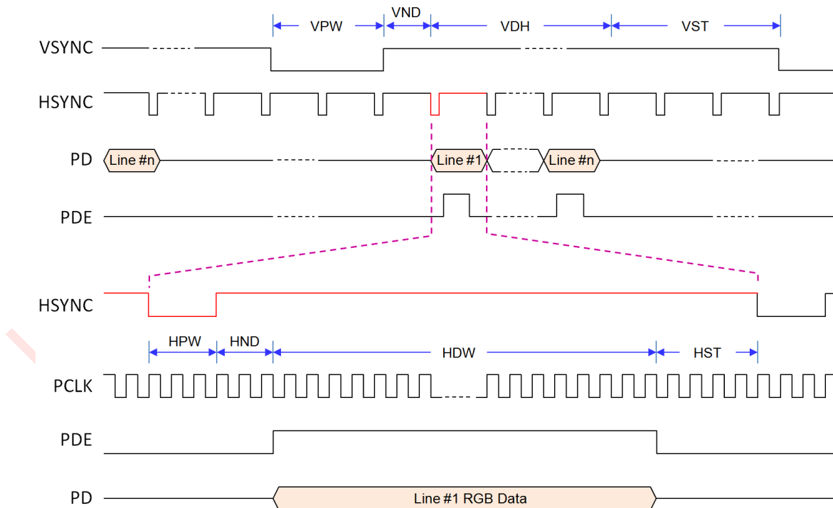
图 7-1: TFT-LCD RGB 接口时序图
