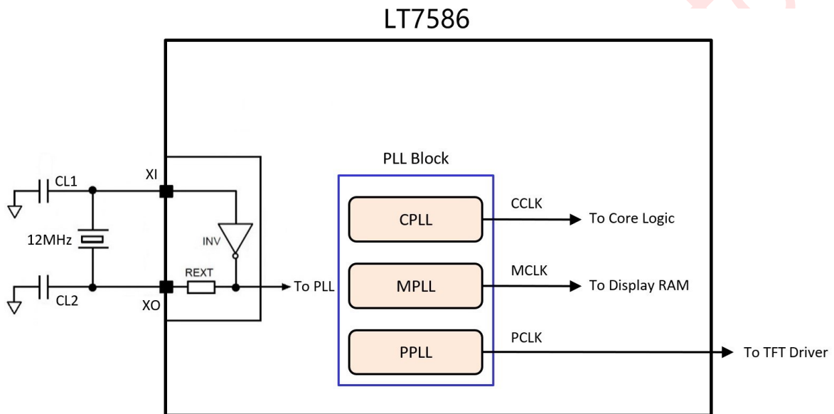
图 4-1: 3 组 PLL 电路
