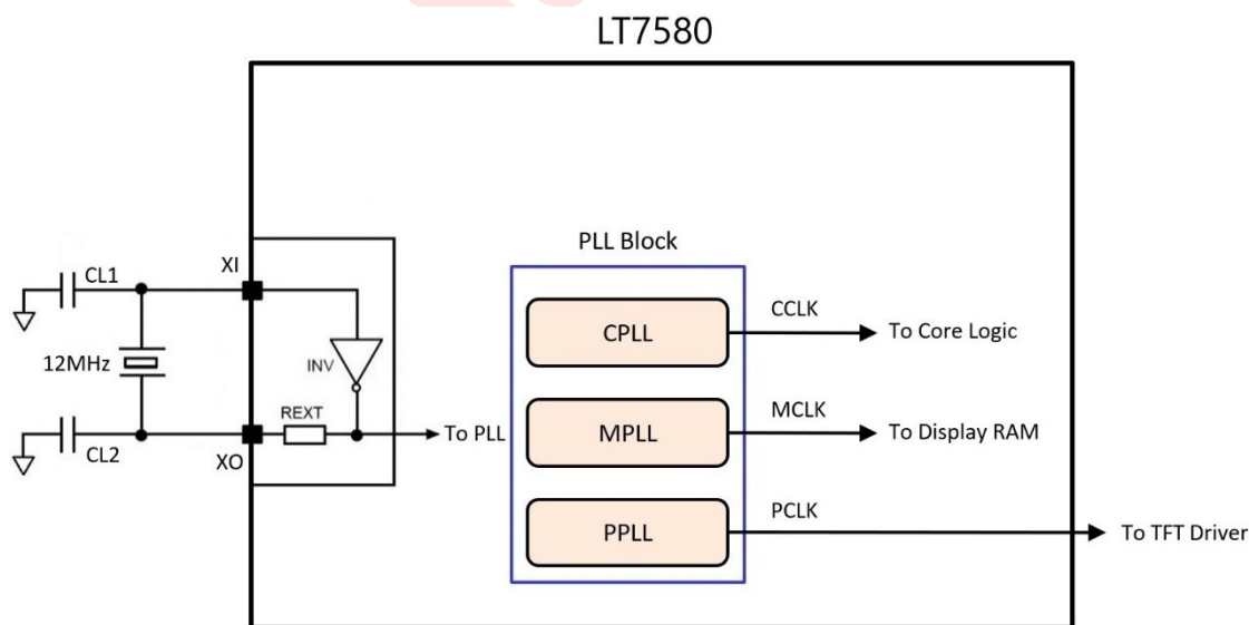
图 4-2：3 组 PLL 电路
