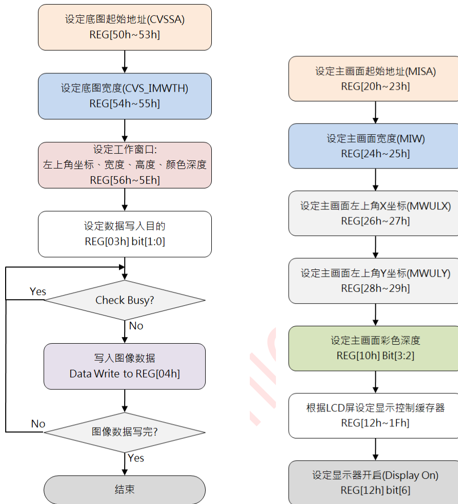
图 8-4：写入及显示主视窗图像
