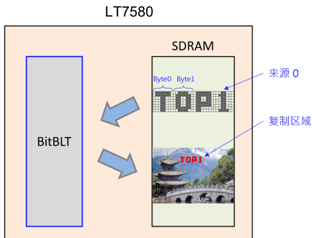
图 10-36: 结合扩展色彩与 Chroma Key 的内存复制范例
