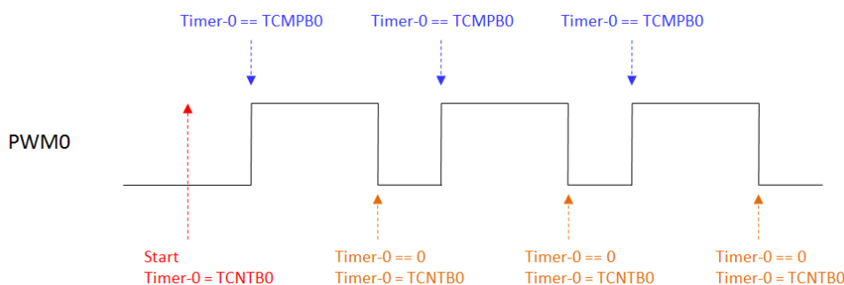
图 12-1: PWM 波形图
