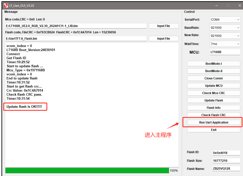
图 2-16: UartTFT-II_Flash.bin 烧录完成
