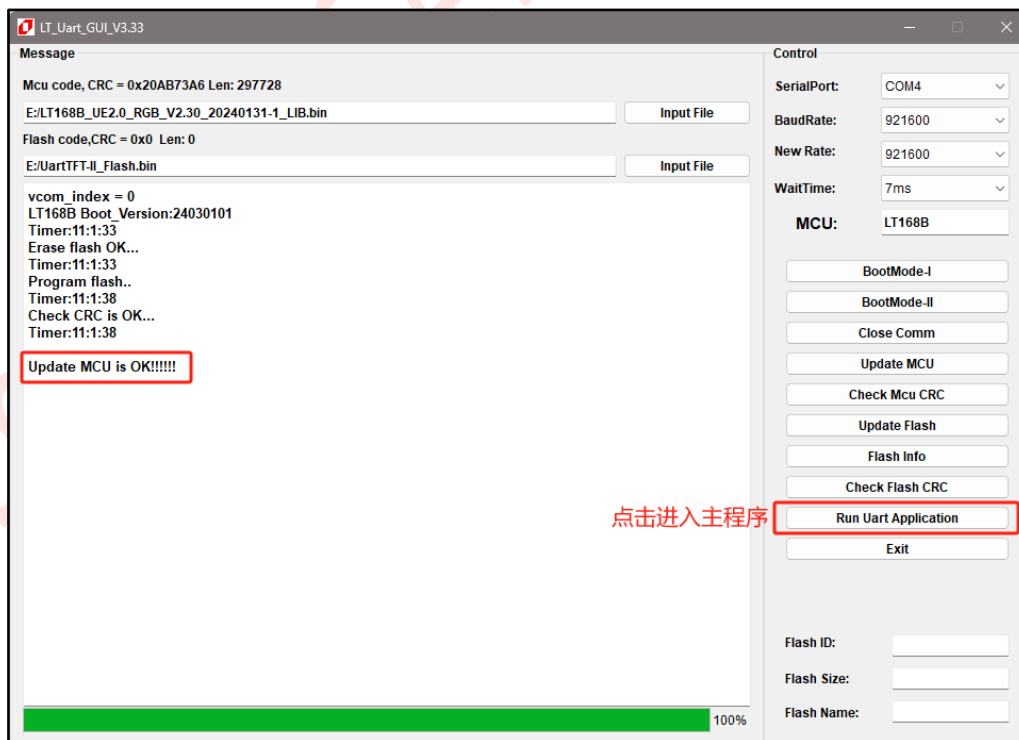
图 2-31：MCU_Code.bin 烧录完成
