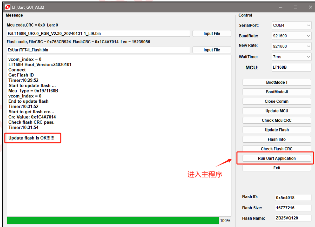
图 2-11：UartTFT-II_Flash.bin 烧录完成
