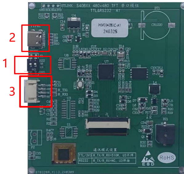
图 2-12：串口更新 UartTFT-II_Flash.bin 接线示意图
