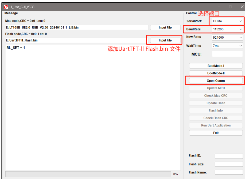
图 2-14: 打开 LT_Uart_GUI 软件点选 UartTFT-II_Flash.bin 及选择连接端口
