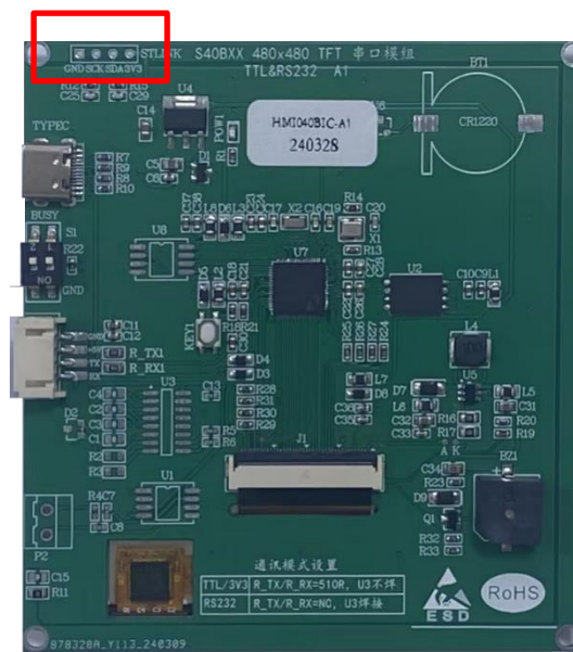
图 4-1：演示模块的 SWD 烧录口
