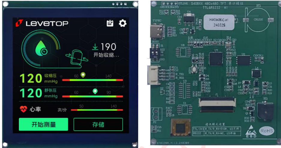
图 1-1: 演示模块外观图
