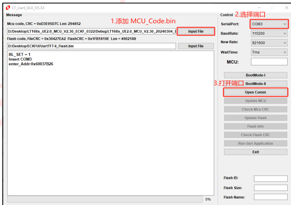
图 2-24: 打开 LT_Uart_GUI 软件点选 MCU_Code 及端口
