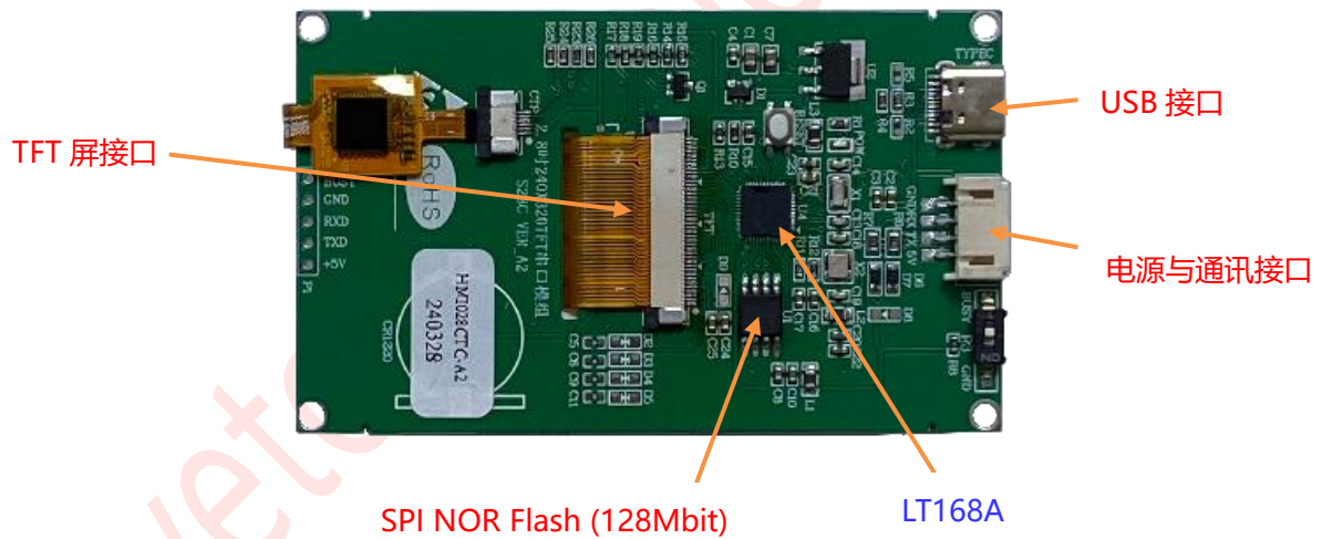
图 1-2: 模块主要组件与接口
