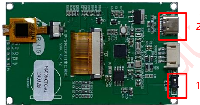
图 2-23: LT168A 接线示意图
