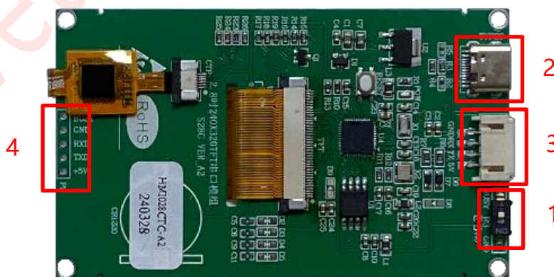
图 2-10: LT168A 接线示意图
