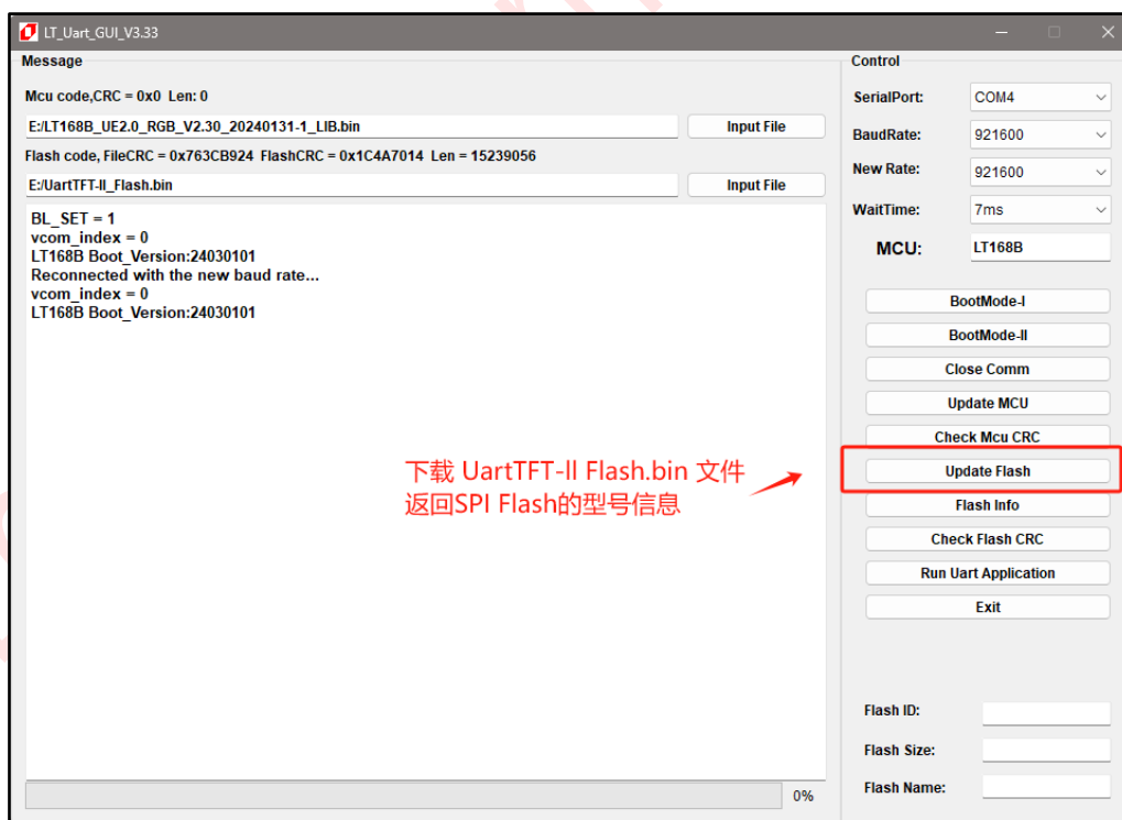
图 2-20: 烧录 UartTFT-II_Flash.bin
