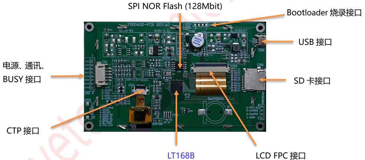
图 1-2: 模块主要组件与接口
