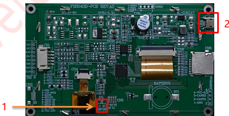
图 2-7: LT168B 接线示意图
