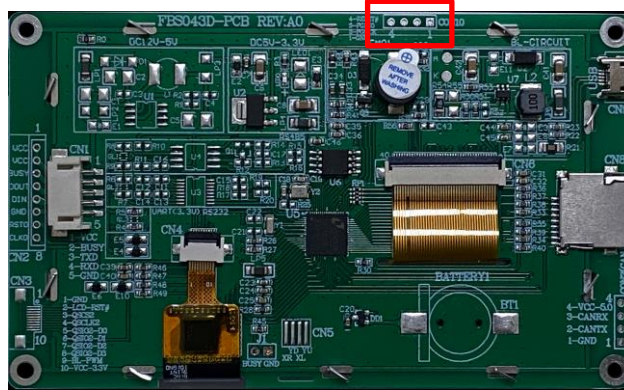
图 4-1：演示模块的 SWD 烧录口
