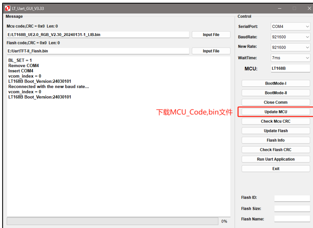
图 2-32：烧录 MCU_Code.bin
