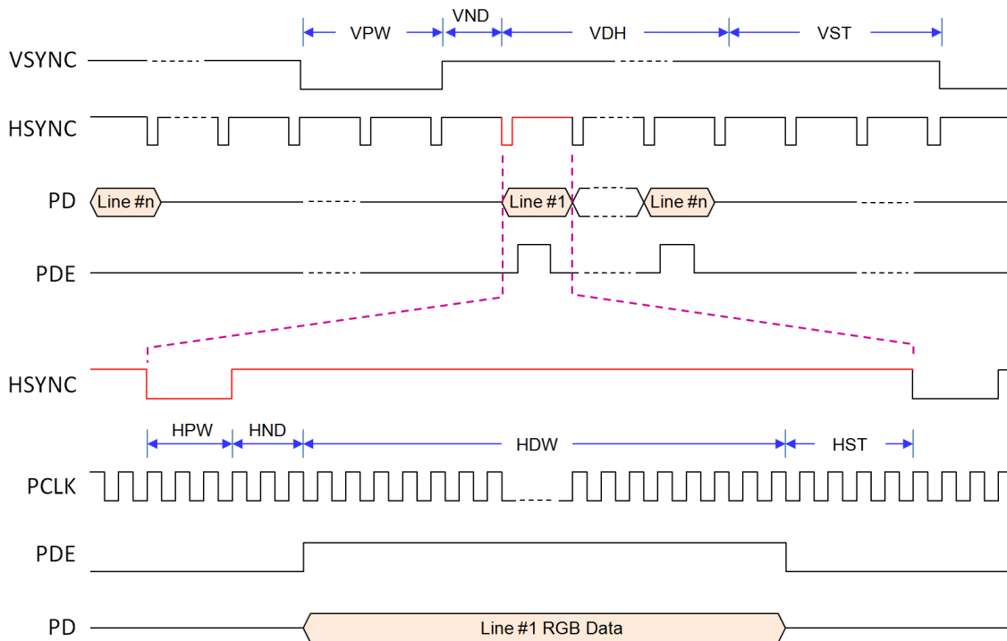
图 12-2: TFT-LCD 接口时序图
