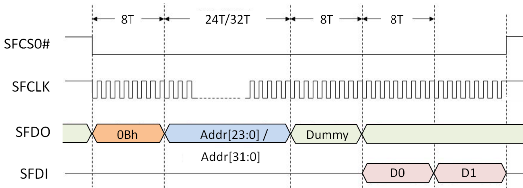
图 17-7: SPI 闪存的快速读取命令
