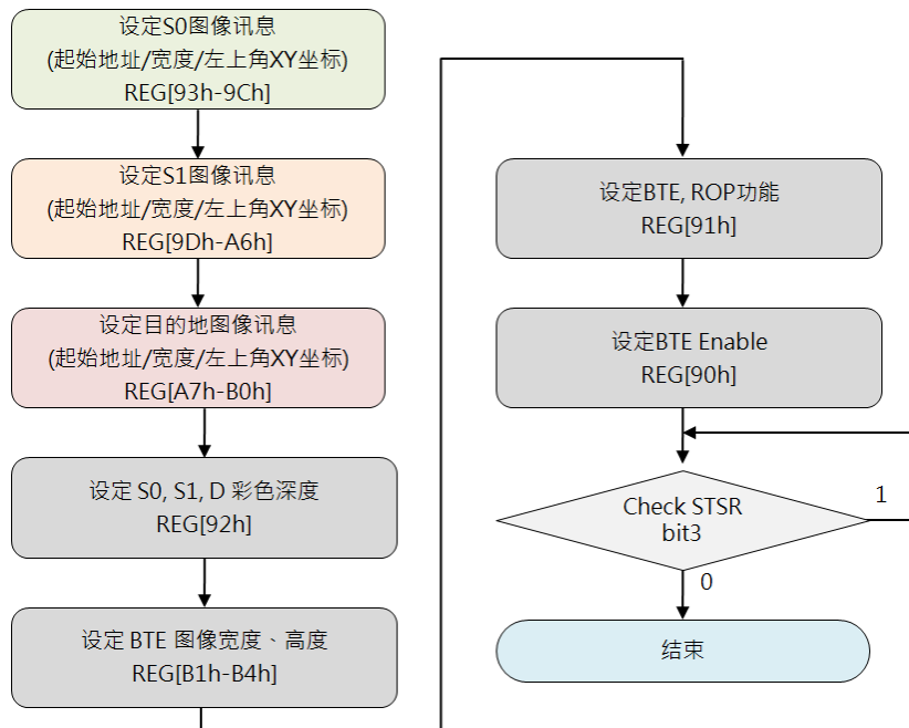
图 15-15: 结合光栅操作的图样填满流程图
