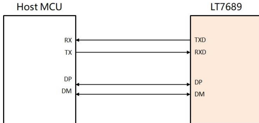
图 10-1: 与主控端 MCU 的通信模式
