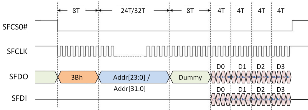
图 17-8: SPI 闪存的读取命令 (数据输入为交错式)
