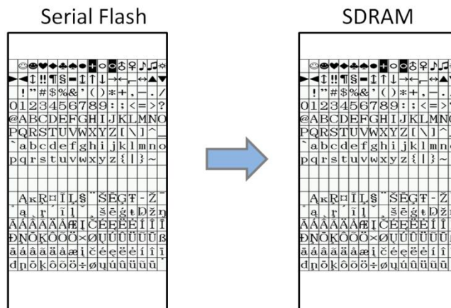
图 17-10: 串行闪存的线性模式 DMA 传输
