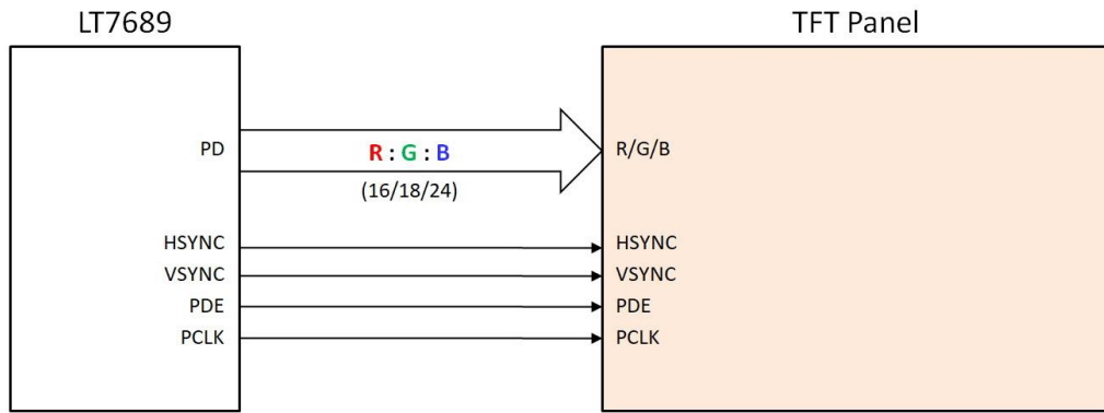
图 12-1: TFT-LCD RGB 接口
