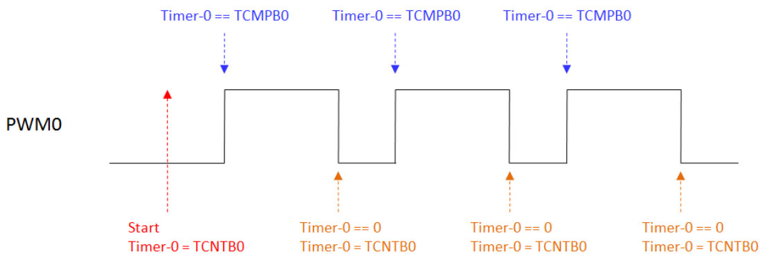
图 10-3: TFT_PWM 波形图
