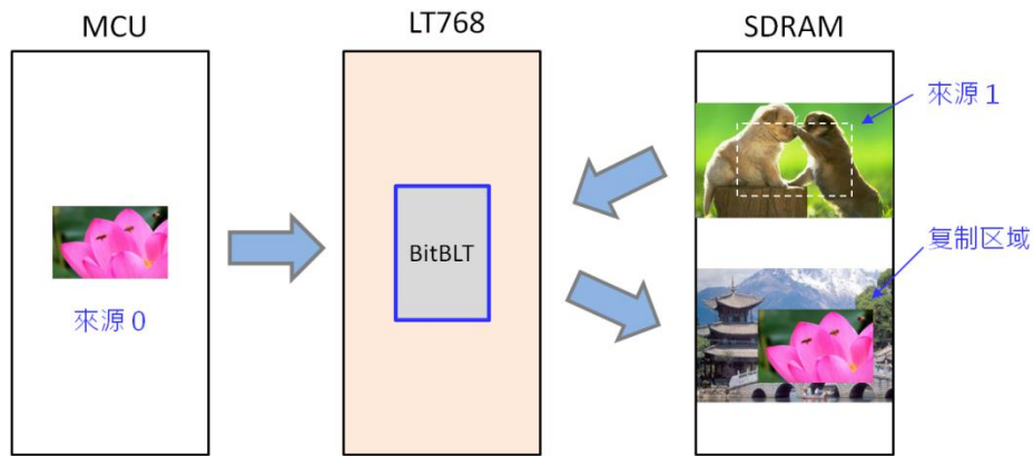
图 15-4: 结合光栅操作的 BTE 写入范例
