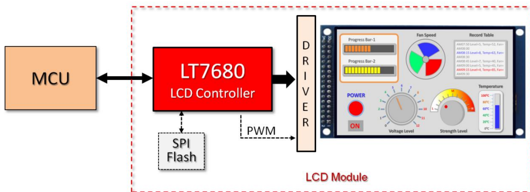
图 1-3: LT7680x-R 设置在 LCD 模块上
