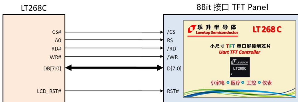
图 8-3: LT268C 与 8 位并口的 MCU 屏连接
