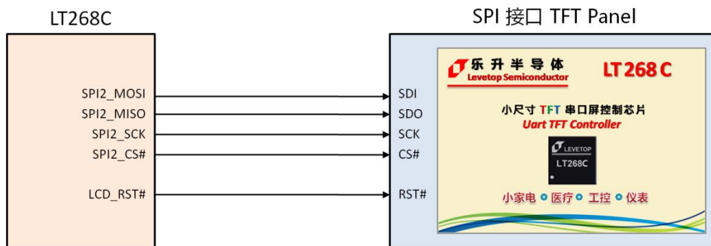
图 8-4: LT268C 与 SPI 接口的 MCU 屏连接
