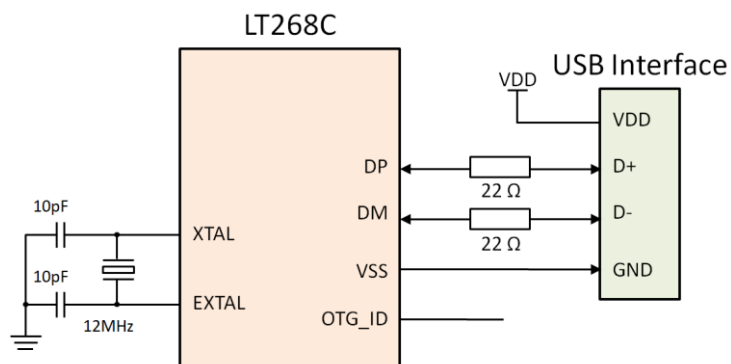
图 8-11: LT268C 连接到 USB 的应用电路
