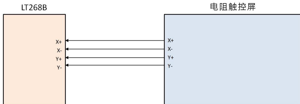
图 8-6：LT268B 连接到电阻式触控屏
