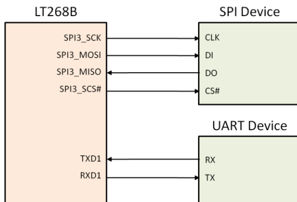
图 8-11：额外的 SPI、SCI 接口参考原理图
