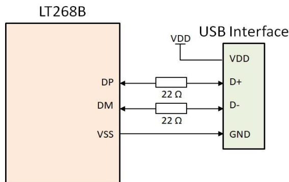
图 8-5 : LT268B 连接到 USB 的应用电路
